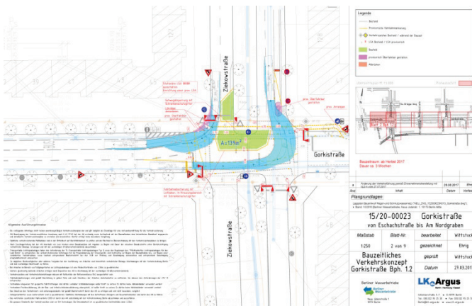
Berlin-Reinickendorf, Gorkistraße: Verkehrsführungsplan mit Darstellung des Baubereichs (grün) und Schleppkurvennachweisen (blau)
