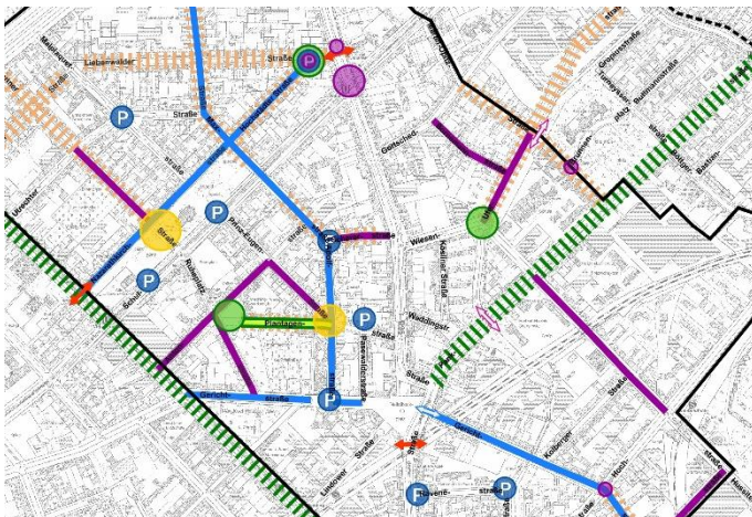
Pankstraße: Integriertes verkehrliches Maßnahmenkonzept (Ausschnitt)
